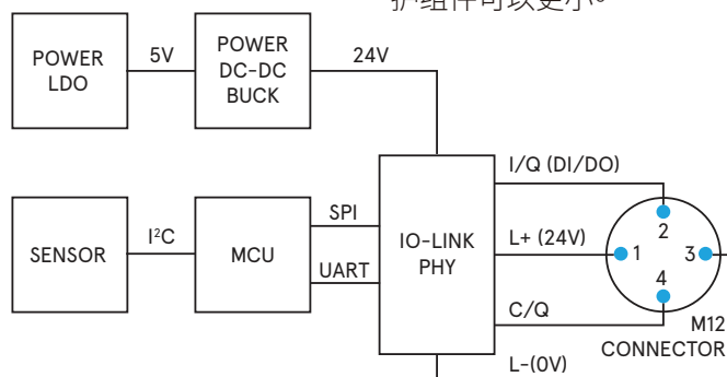
图 2. IO-Link 传感器的构建块
