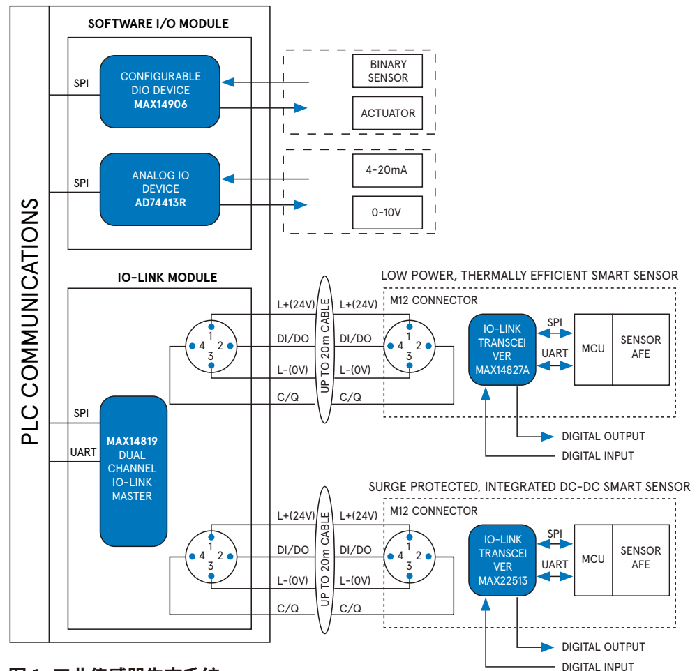
图 1. 工业传感器生态系统
